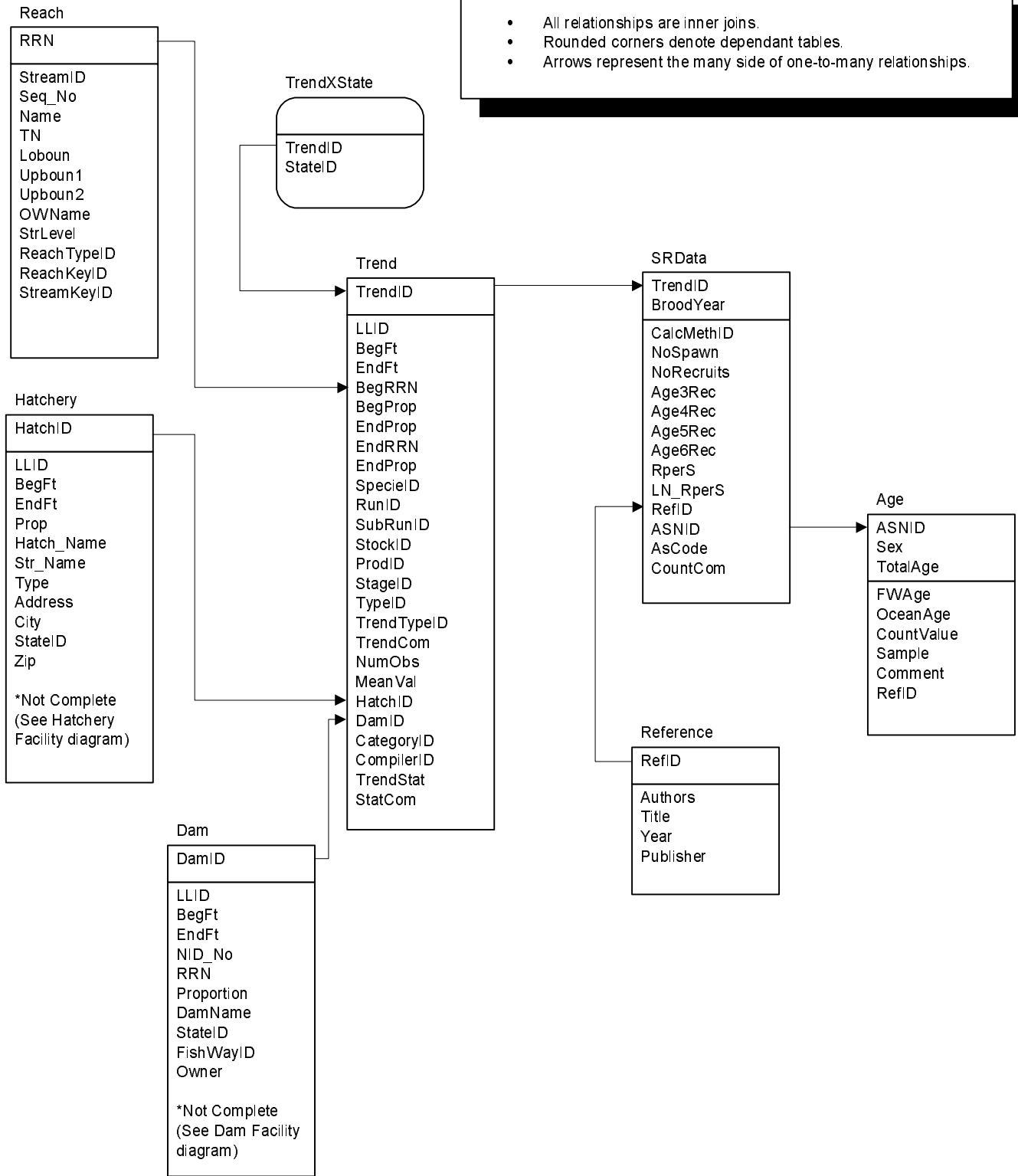
Figure 1. ER diagram for SR Data.
